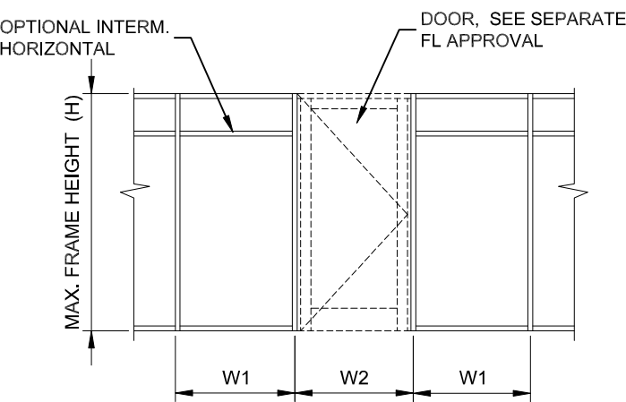
ELEVATION E4
