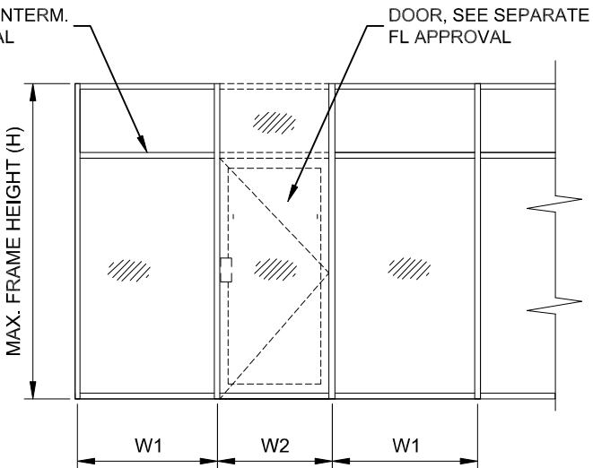
ELEVATION E3
