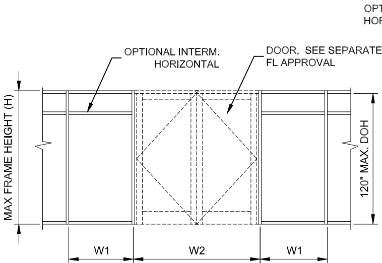
ELEVATION E2
