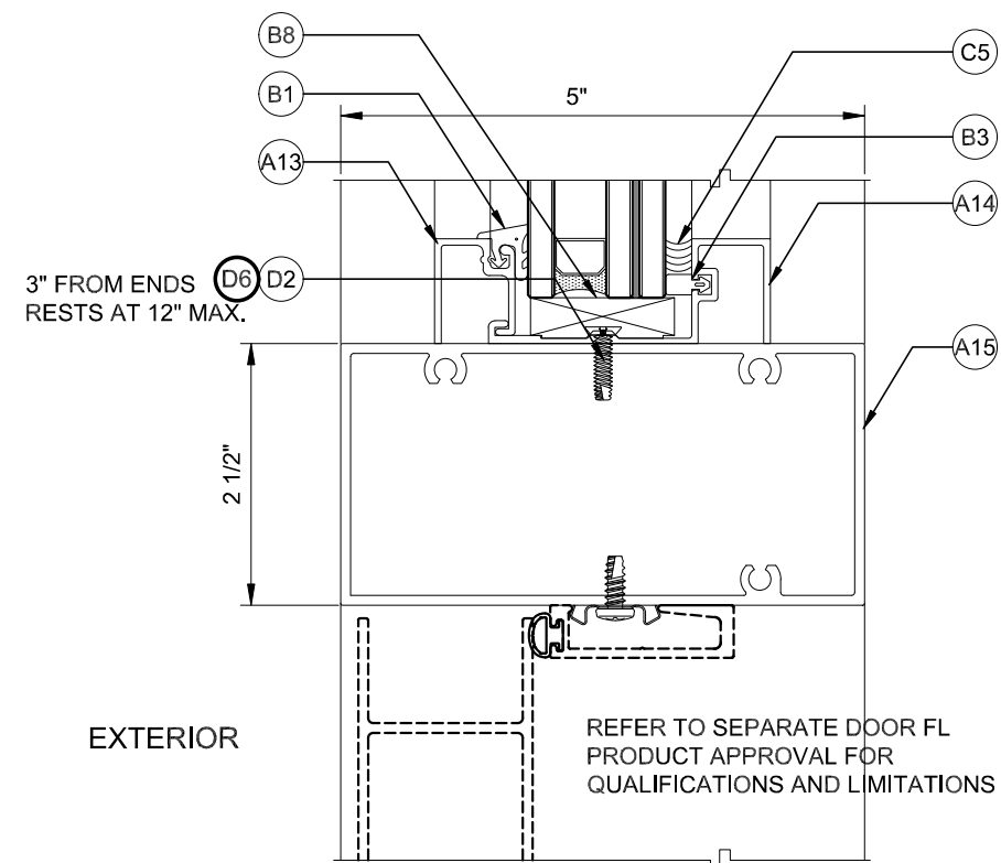
3 DOOR TRANSOM DETAIL
