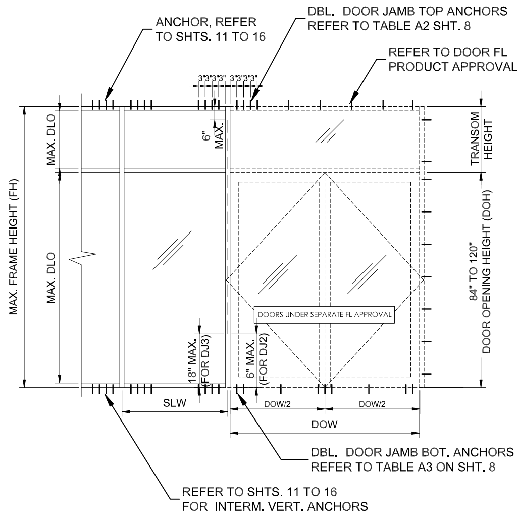
ELEVATION E5
