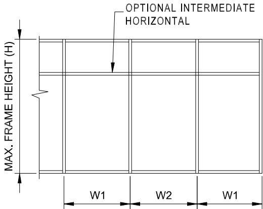
ELEVATION E1
